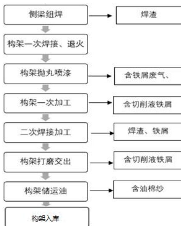
图4.2-3 构架生产工艺流程
