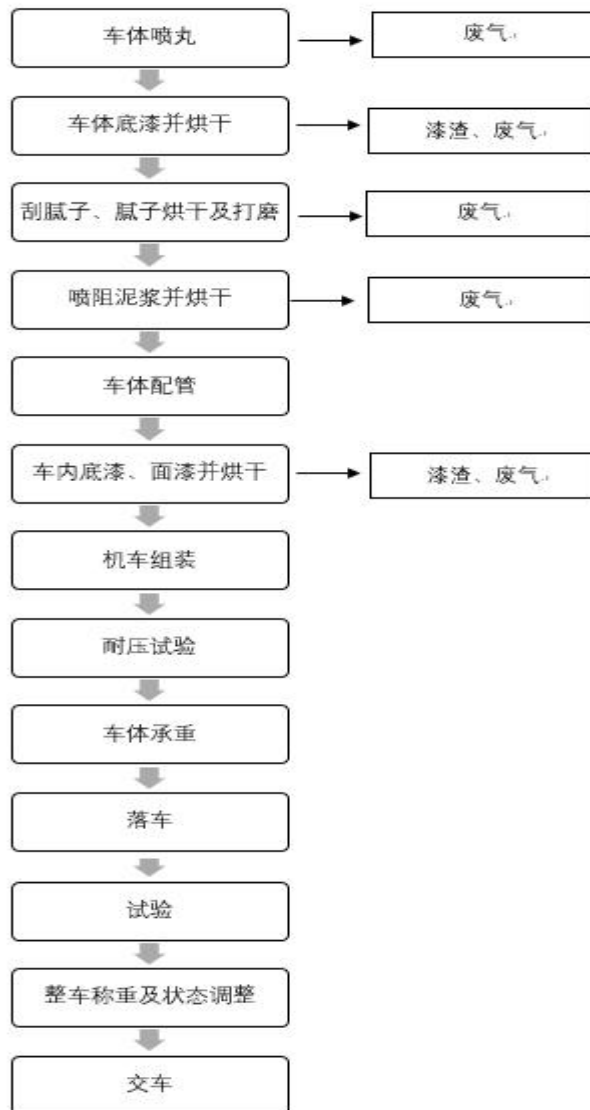
图4.2-2 机车组装及试验工艺流程
