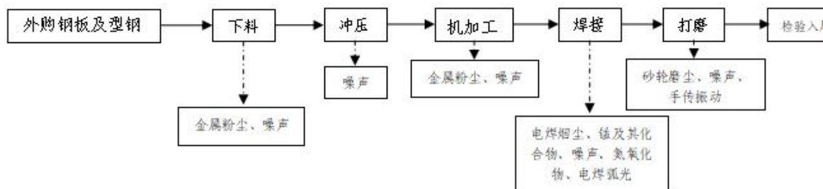
图4.2-6 机车配件生产工艺流程图
